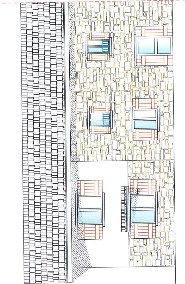
PROSPETTO SUD scala 1:100
